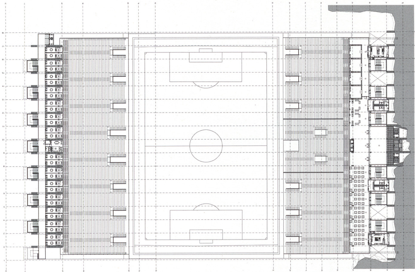
PLANTA ZONA VIP Y CAMAROTES
