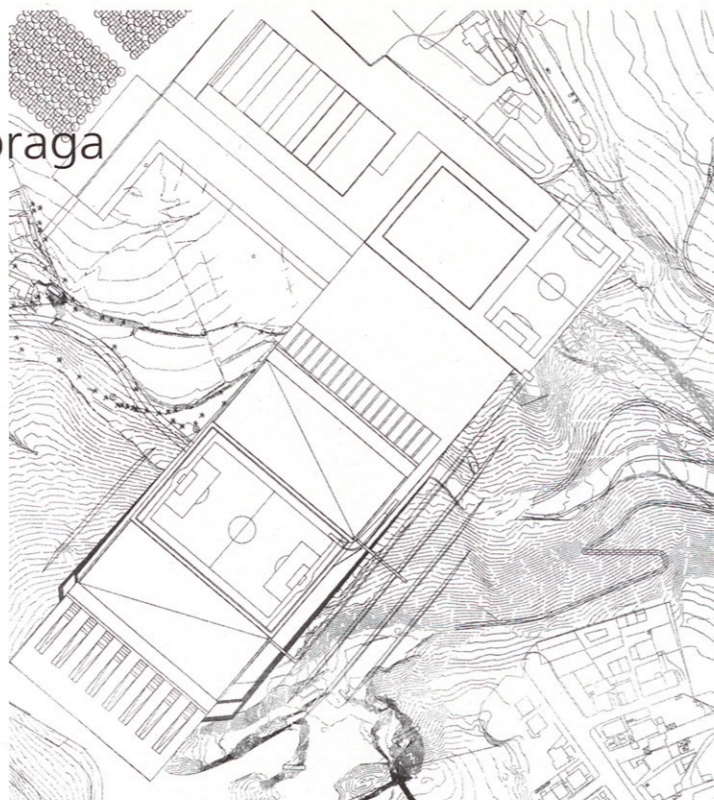
PLANTA DE SITUACIÓN
