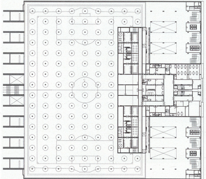
PLANTA SÓTANO
